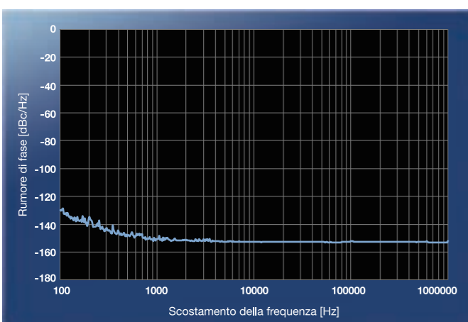
Rumore di fase TX (banda 14 MHz, Modalità: CW)
