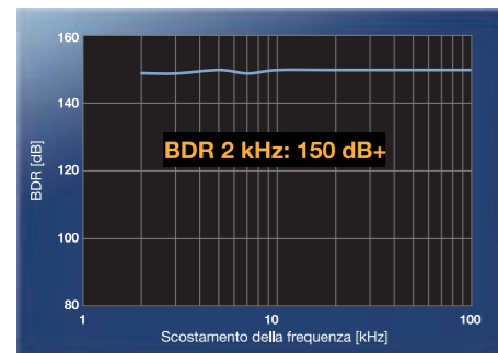
14 MHz Gamma dinamica di blocco Gamma dinamica (BDR)
