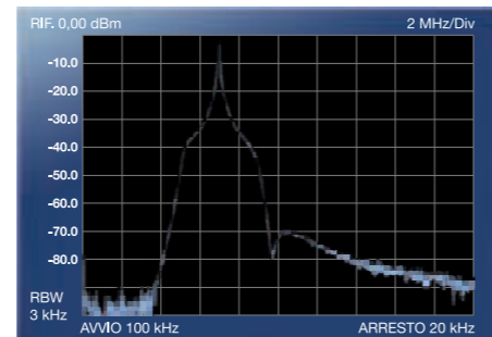
VC-Tune + filtro passabanda (7 MHz, intervallo 20 MHz)
