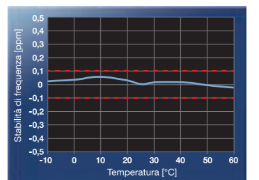
Stabilità in funzione della temperatura del TCXO
