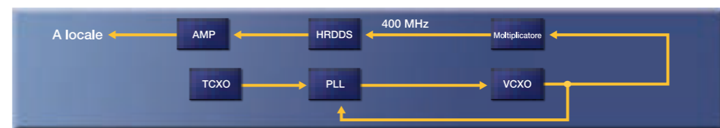
Schema a blocchi del circuito locale
