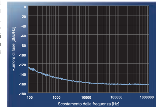
Rumore di fase 1° oscillatore locale (14.2 MHz)
