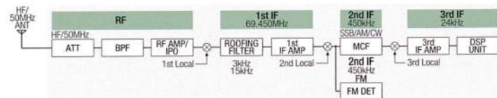
Schema a blocchi del ricevitore
