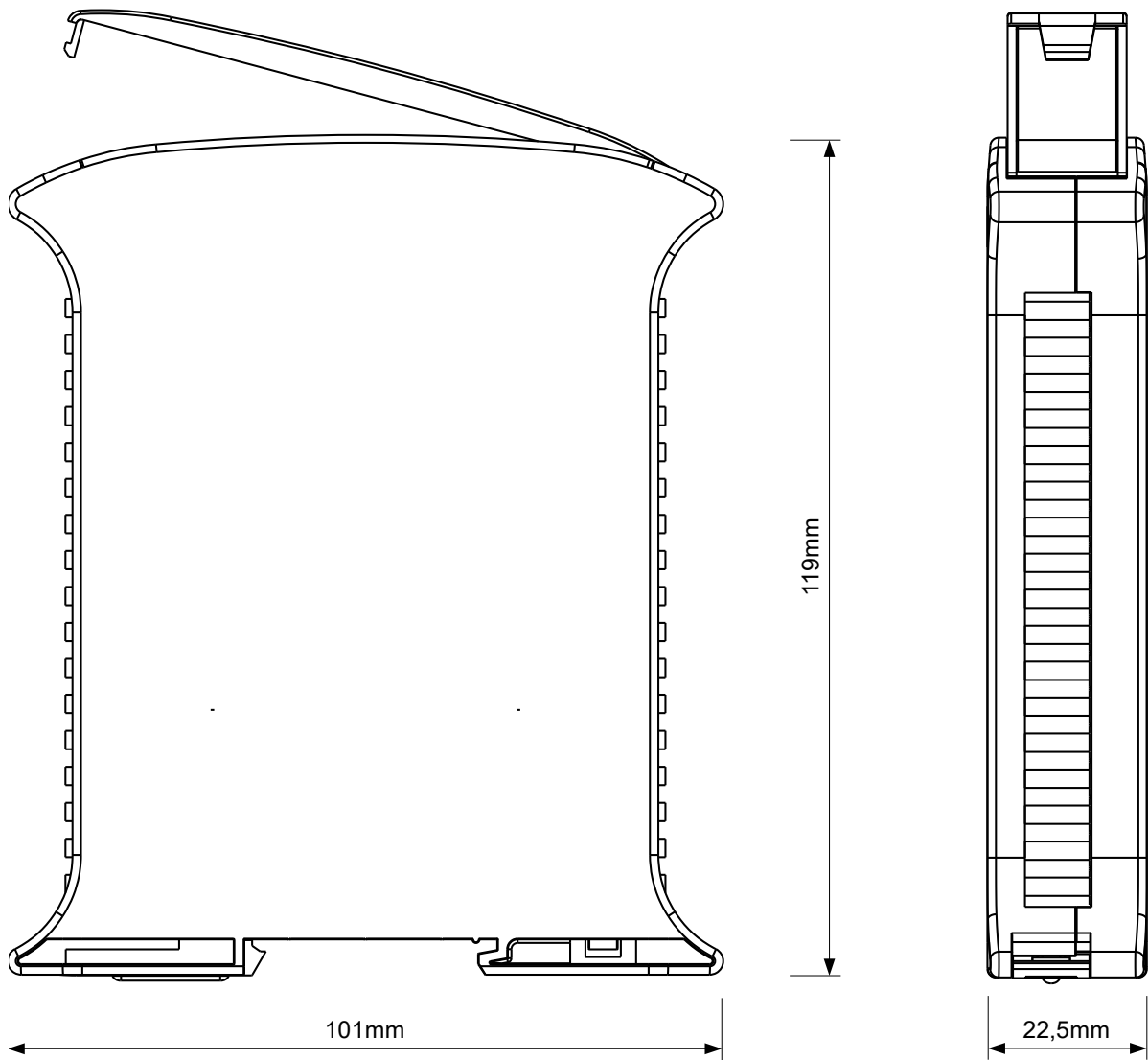
Figura 2: Ingombri meccanici
