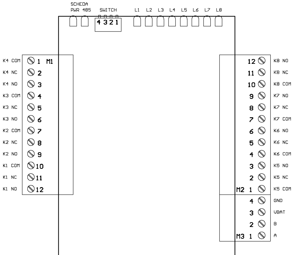
Figura 3: Posizione e numero dei terminali
